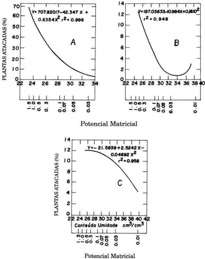
Figura 1. Relação entre a percentagem de plantas de milho atacadas pela lagarta Elasmopalpus lignosellus com quatro (A), 10 (B) e 15 (C) dias de idade e o conteúdo de umidade potencial matricial de um Latossolo Vermelho Escuro, CNPMS, Sete Lagoas, MG, 1992.
